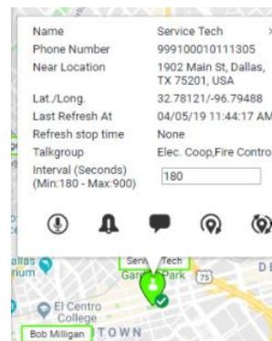
Details Teilnehmer
