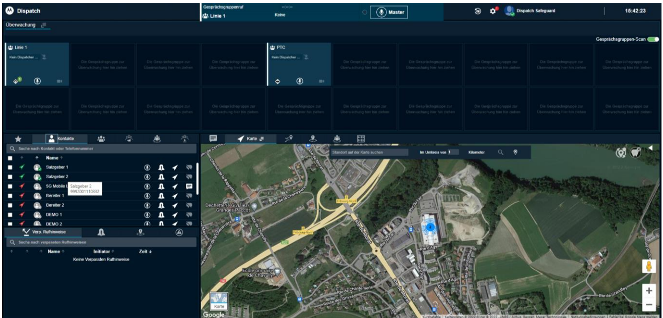
Hauptansicht Dispatch
