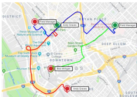
Ansicht Standortverlauf
